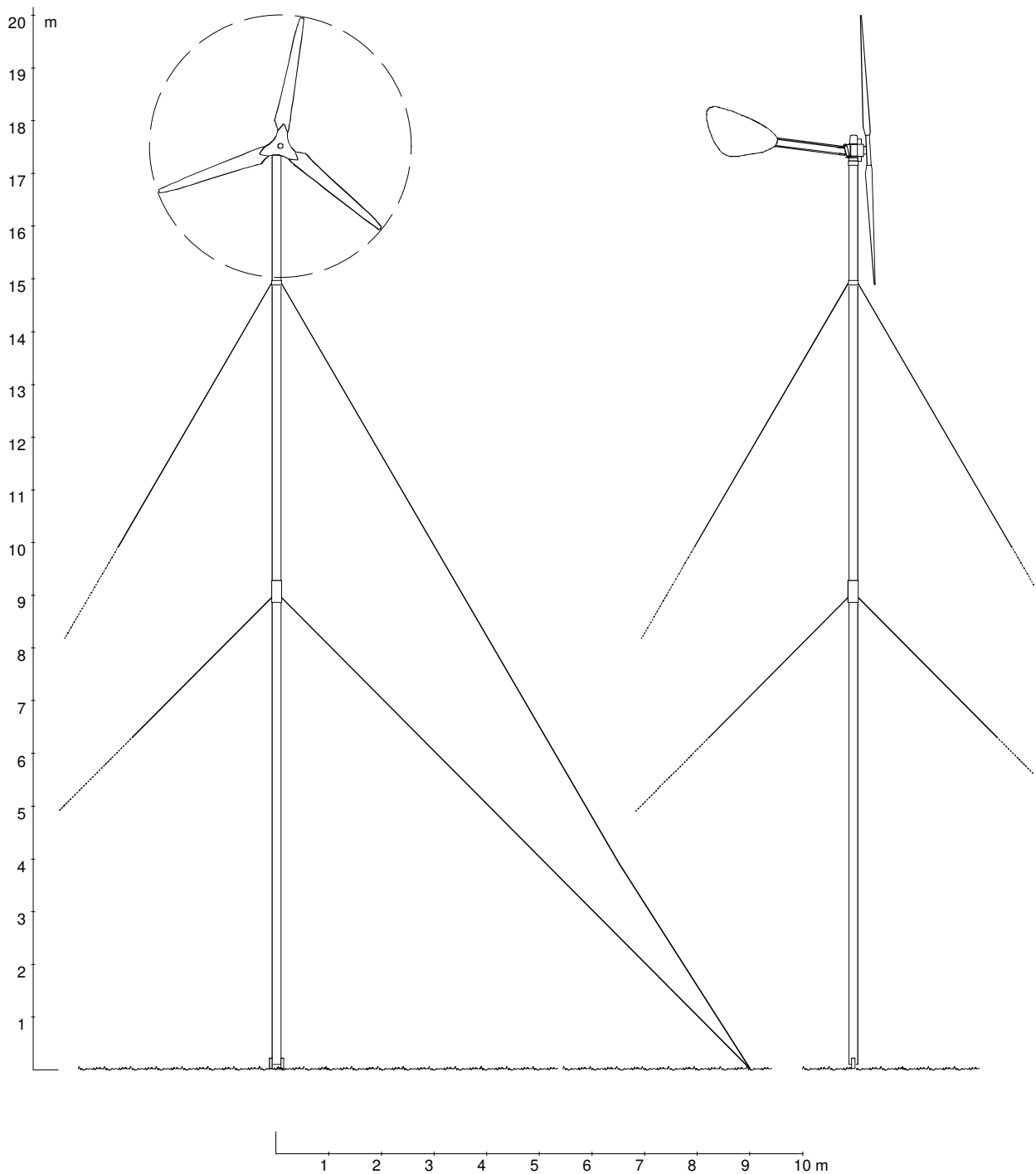
TuuleT188 tuulivoimala edestä ja sivulta nähtynä Mittakaava 1:100
